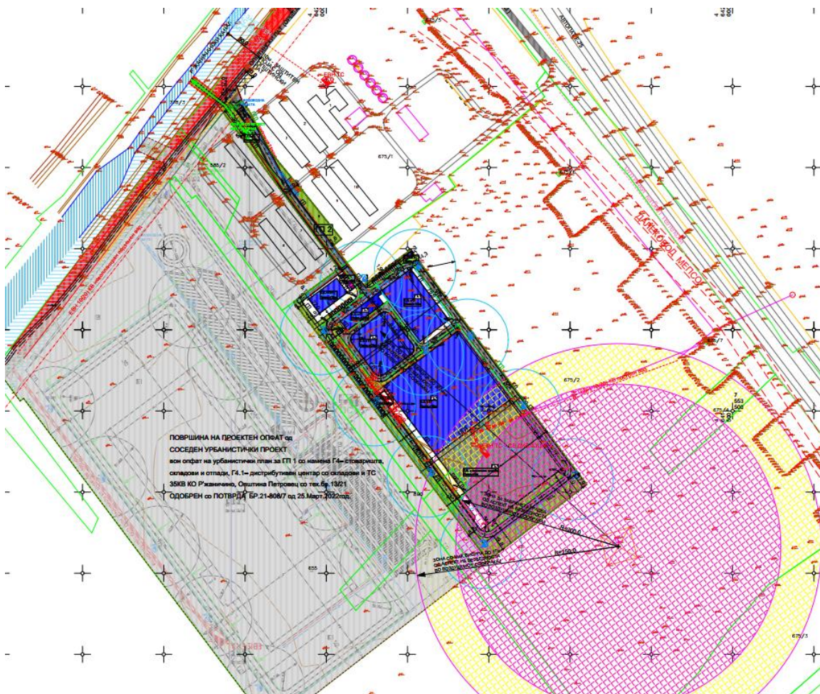
Графички приказ за Урбанистичкиот проект вон опфат на урбанистички план за ГП 2 со намена Г3-производство на енергија од обновливи извори, Г3.7 - биогазна централа од 3MW, КО Р'жаничино, Општина Петровец
